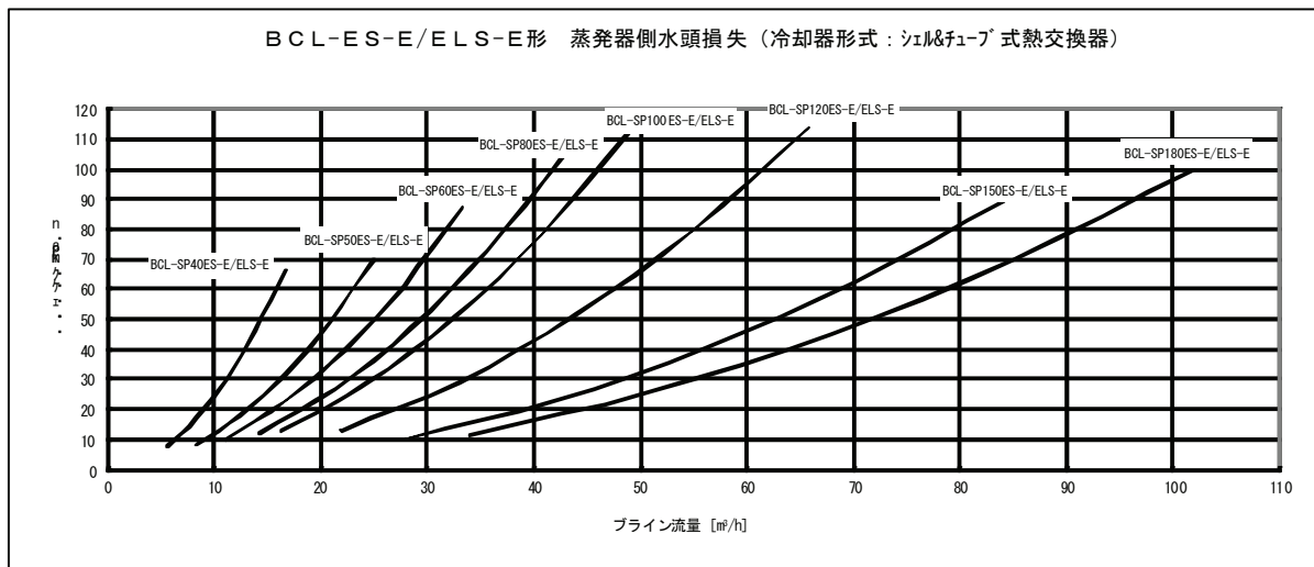
図 3-2 蒸発器側水頭損失
