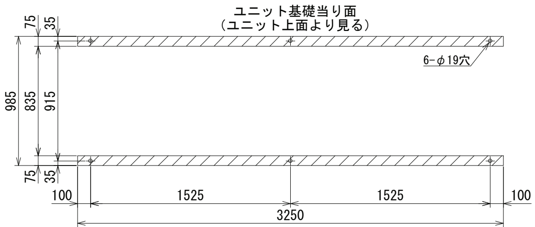
図 2-2 基礎図
