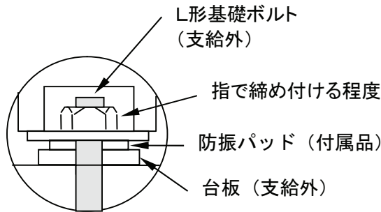
図 2-4 防振パッド取付要領
