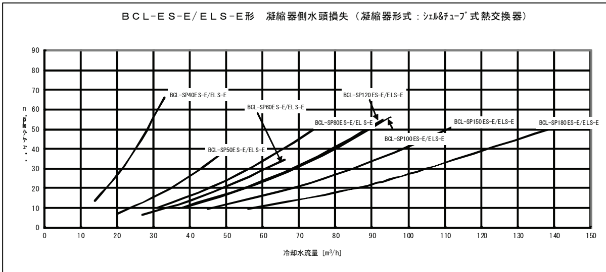
図 3-1 凝縮器側水頭損失
