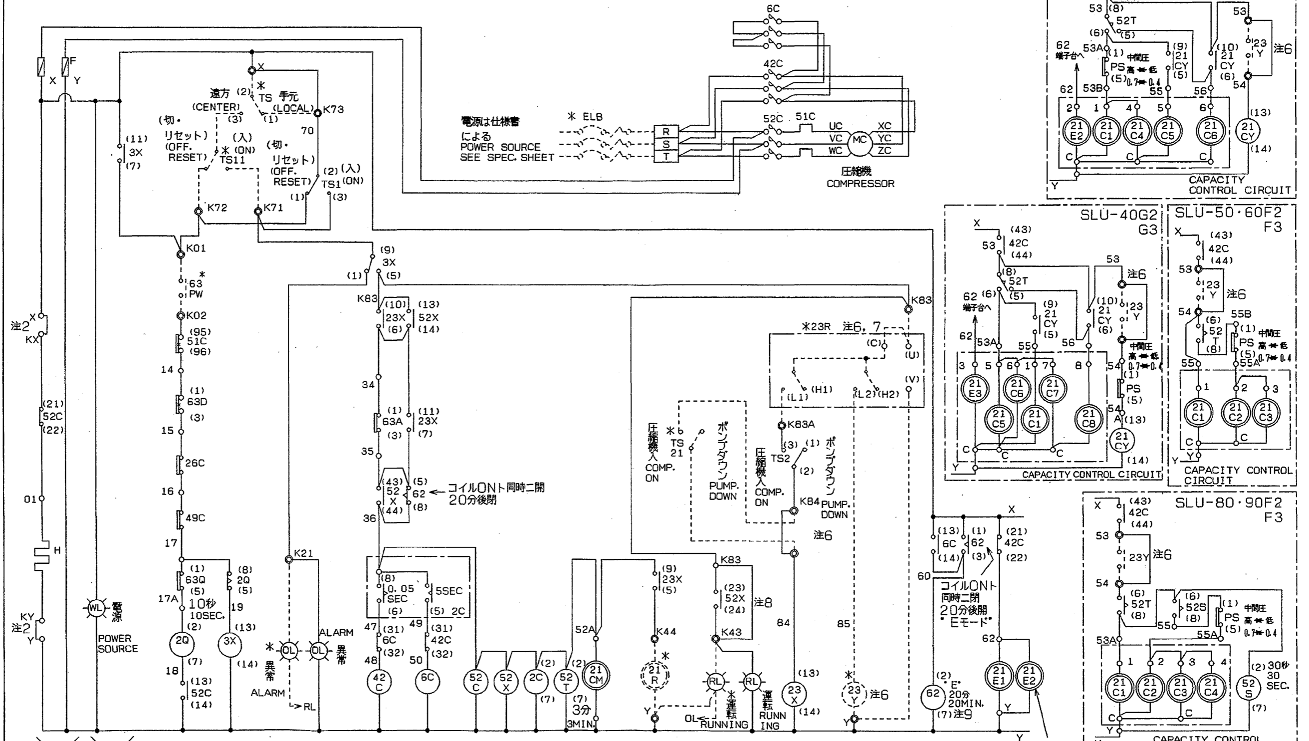
クランクケース 電源表示 HEATER CIRCUIT POWER SOURCE INDICATION 運転指令・保護回路 異常表示 RUNNING SIGNAL PROTECT CIRCUIT ALARM INDICATION 圧縮機運転回路 (入-△) COMP. RUNNING CIRCUIT 液ライン LIQUID LINE 運転表示 RUNNING サーモ (発停) THERMOSTAT 再始動制限回路 RESTARTING RESTRICTED CIRCUIT 均圧回路 EQUALIZING CIRCUIT
