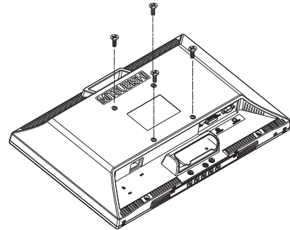
【VESA穴ネジの取外し】
