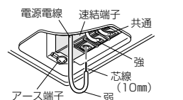
※単一風量機種は弱の箇所には差し込み口はありません。上図の共通・強の差し込み口に電源電線を差し込みます。
