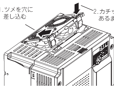
FR-F720PJ-5.5K-FSの例
