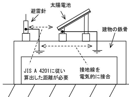
図表 6. 太陽電池モジュールと避雷設備の絶縁距離および接地構造
