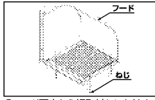
①フード下方から網取付ねじを外す。
