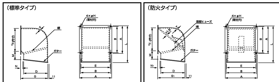
外形寸法表 (単位:mm)
