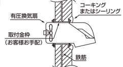
断面図
