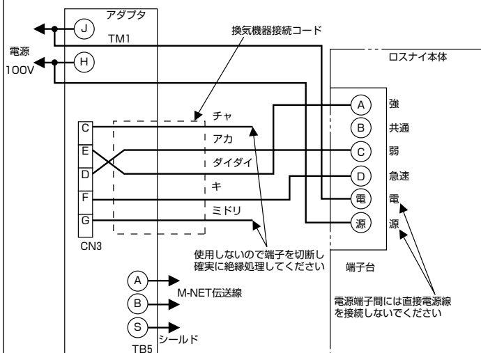
結線図 9
