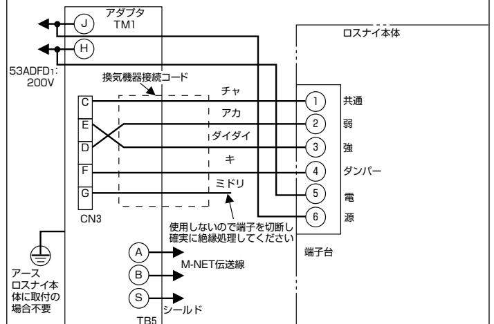
結線図 4
