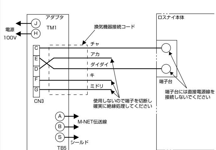
結線図 7
