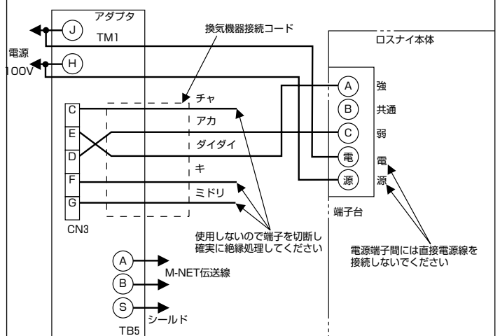
結線図 8
