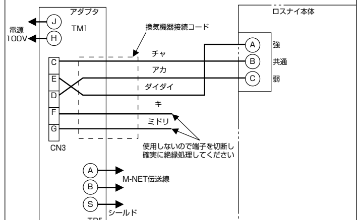
結線図 6
