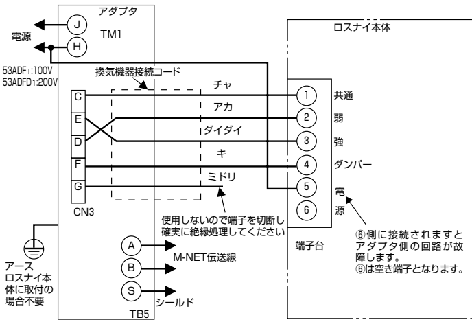
結線図 3
