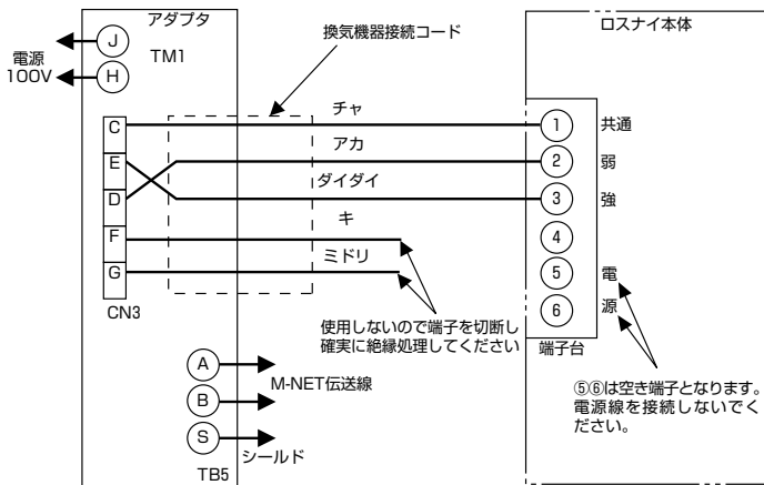
結線図 5
