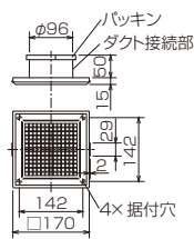
副吸込グリル(同梱品)
