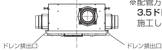
②正面図
