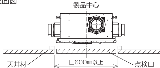
②正面図
