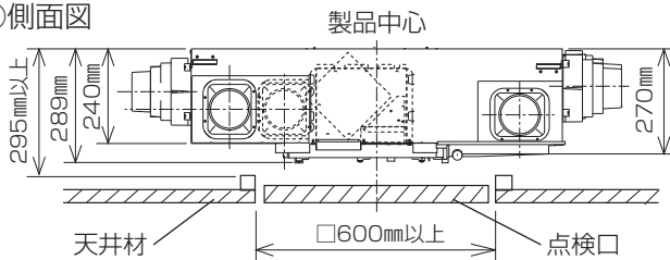
①側面図
