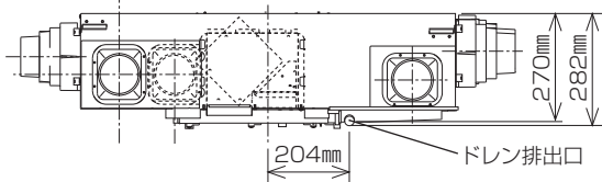
①側面図
