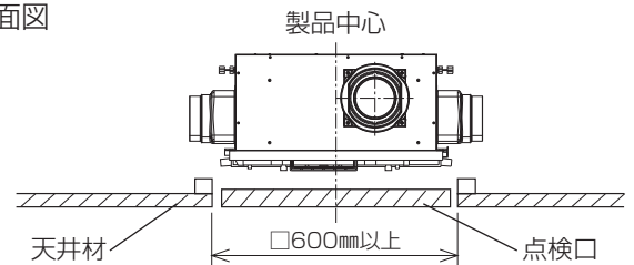
②正面図
