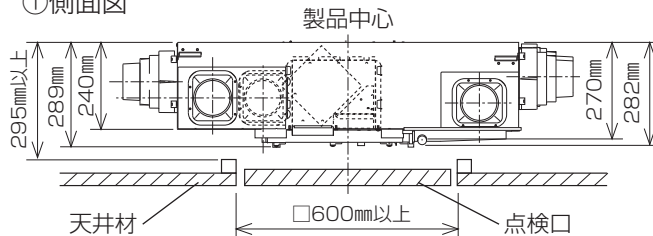
①側面図
