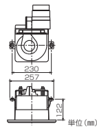
天吊金具 P-02TK (別売システム部材) 据付位置 (2点吊り)
