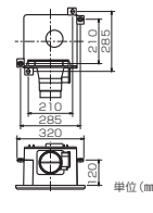
天吊金具 P-04TK (別売システム部材) 据付位置 (2点吊り)
