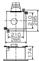
天吊金具P-05TKタイプ （別売システム部材） 据付位置（2点吊り） 単位(mm)
