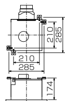
天井金具P-05TKタイプ （別売システム部材） 据付位置（2点吊り） 単位（mm）
