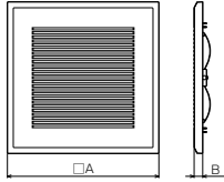
■インテリア格子 (-C, -CB, -CK, -G, -GV) タイプ
