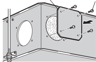
フランジカバー 取付ねじ (フランジカバー用)
