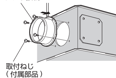
ダクト接続フランジ
