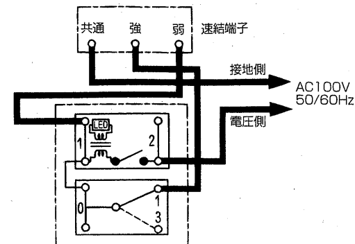
コントロールスイッチ(P-03CSLs)システム部材
