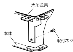
天吊金具P-05TKタイプ (別売システム部材) 据付位置(2点吊り)
