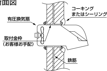
断面図
