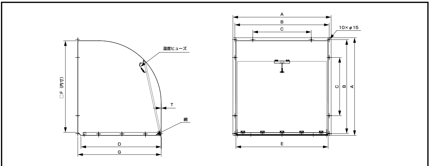
外形寸法表
