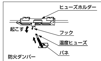
④防火ダンパーを支えたまま、フードのヒューズホルダーは防火ダンパーを載せるように起こし、バネにひっかけた温度ヒューズをフックに近付ける。
