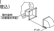
取付図
