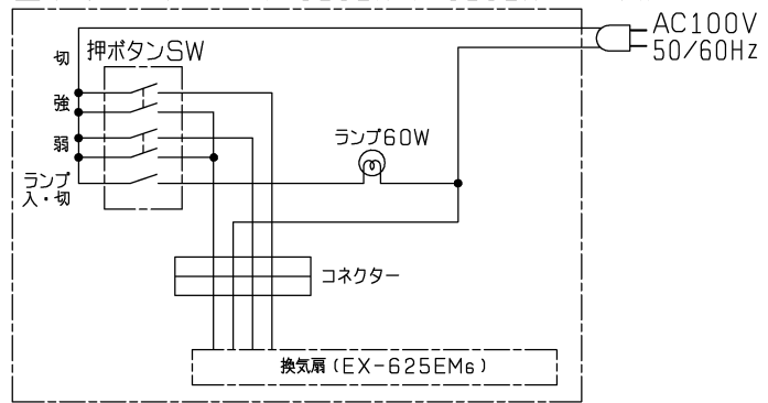
キッチンフード本体 (V-625EH, V-625EH 2 )
