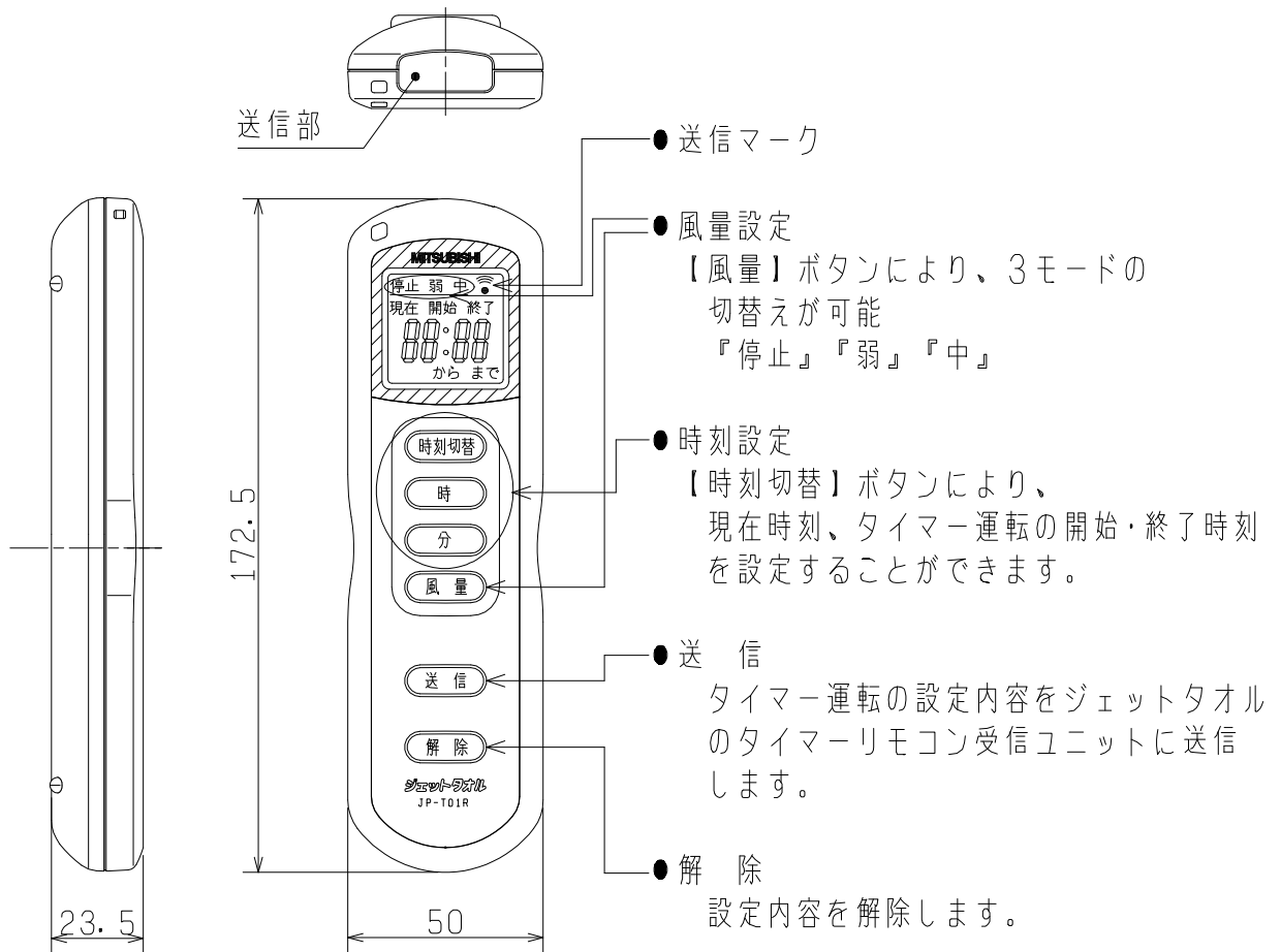
■タイマーリモコン運転モード時の騒音 単位 (dB)
