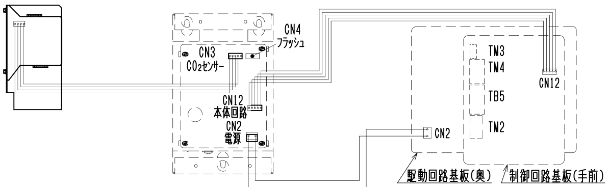
CO 2 センサー (基板部)
