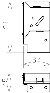
CO 2 センサー (センサー部)
