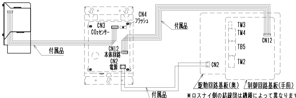
CO 2 センサー (基板部)
