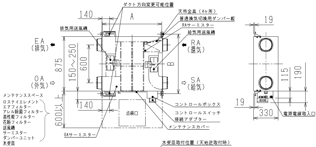
リリース対象機種天吊ボルトピッチ
