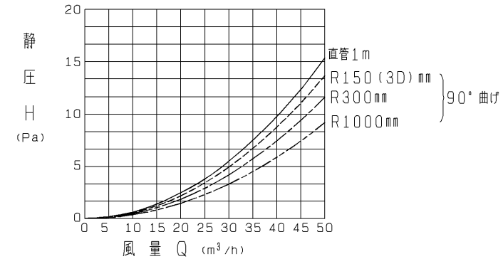
圧力損失特性
