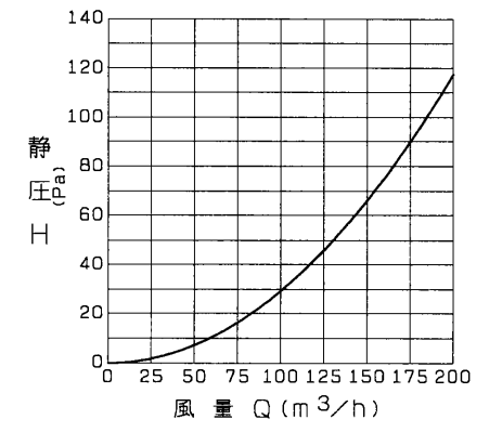
圧力損失特性 (VP, VU管使用時)
