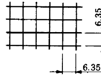
■ 金網詳細図
