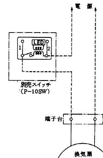
■ 結線図
