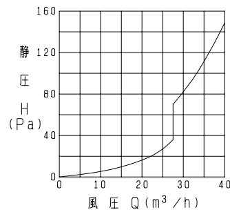
■ 圧力損失特性
