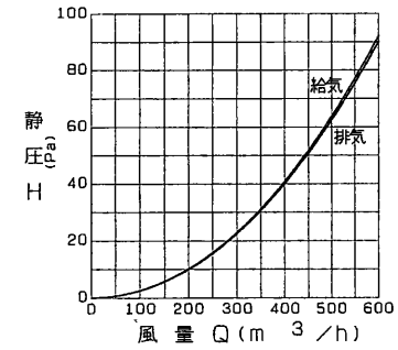
P-18NV 圧力損失特性
