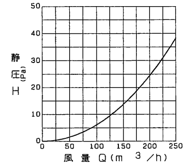
P-13NV 圧力損失特性
