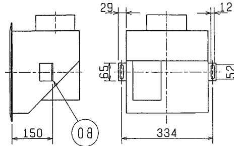
■ 天吊金具取付要領図
