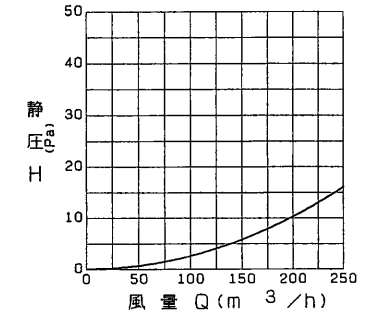
P-15NV 圧力損失特性
