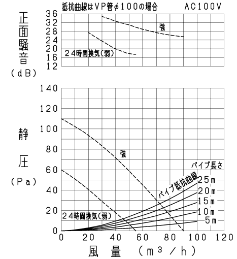
VD-10ZLC 13 -IN/P-Q・騒音特性
