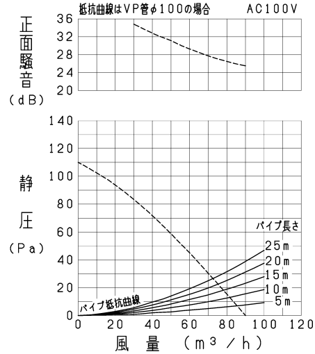
VD-10ZC 13 -IN/P-Q・騒音特性
