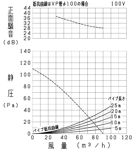
VD-10Z 13 -IN/P-Q・騒音特性
