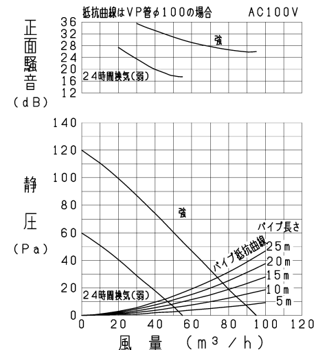
VD-10ZLC 13 -IN/P-Q・騒音特性
