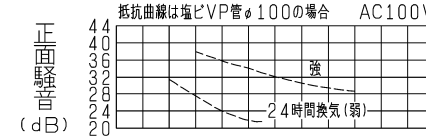
VD-10ZLC 10 -IN/P-Q・騒音特性
