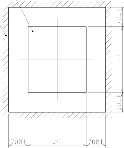
本体取付用 アルミパネル加工寸法
