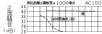
VD-15ZLXP 9 -IN/P-Q・騒音特性
