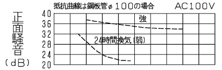
VD-15ZLX 9 -IN/P-Q・騒音特性
