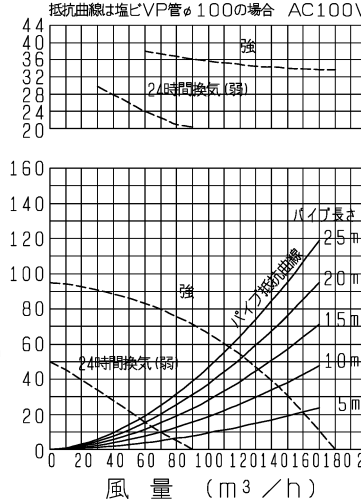
VD-15ZLC 9 -IN/P-Q・騒音特性
