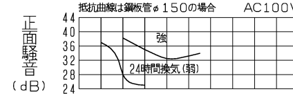
VD-18ZLX 9 -IN/P-Q・騒音特性
