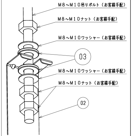
■天吊金具据付図
