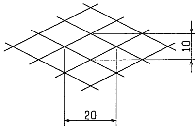
金網拡大図(1:1)
