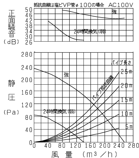
VD-18ZLSC 9 -IN/P-Q・騒音特性
