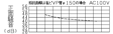
VD-20ZB 9 -IN/P-Q・騒音特性
