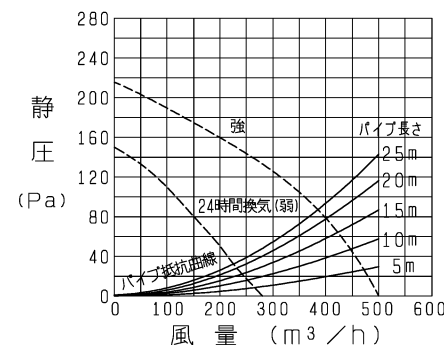
VD-18ZB 9 -IN/P-Q・騒音特性
