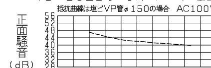
VD-20ZB 9 -IN/P-Q・騒音特性
