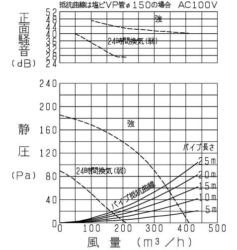
VD-20ZLC 9 -IN/P-Q・騒音特性
