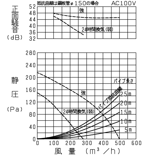
VD-20ZLXP 10 -IN/P-Q・騒音特性
