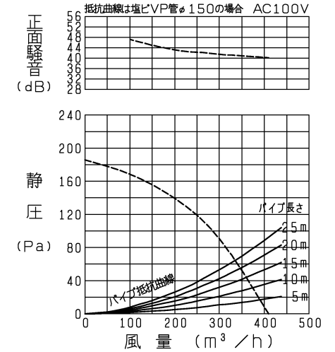
VD-20ZB 10 -IN/P-Q・騒音特性
