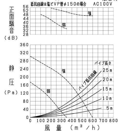
VD-23ZB 13 -IN/P-Q・騒音特性
