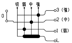
风量切换スイッチの接点状態
