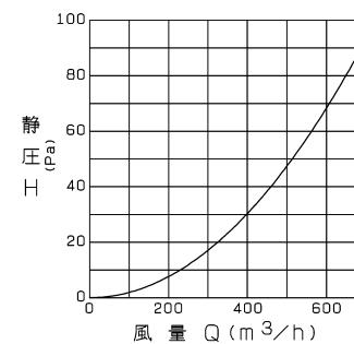
圧損特性
