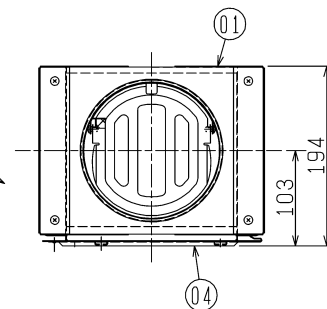
■ 取付板組合せ寸法
