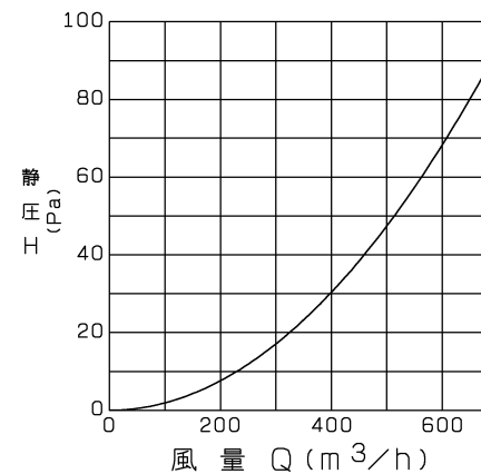
圧力損失特性
